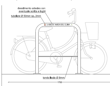
TIPO 1 Stallo portabici ad U rovescio TASSELLATO
