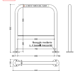
TIPO 1 Stallo portabici ad U rovescio TASSELLATO
