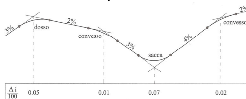
Esempio di profilo altimetrico con i raccordi verticali. Il parametro \Delta i/100 è la variazione di pendenza in percento delle livellette da raccordare (fonte DM 05.11.2001 fig. 5.3.2.a).
