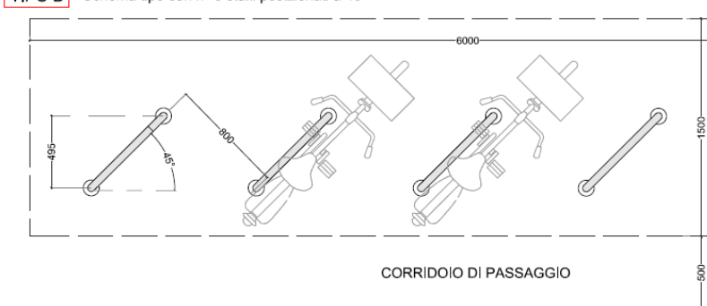
TIPO B Schema tipo con n° 5 stalli posizionati a 45°
