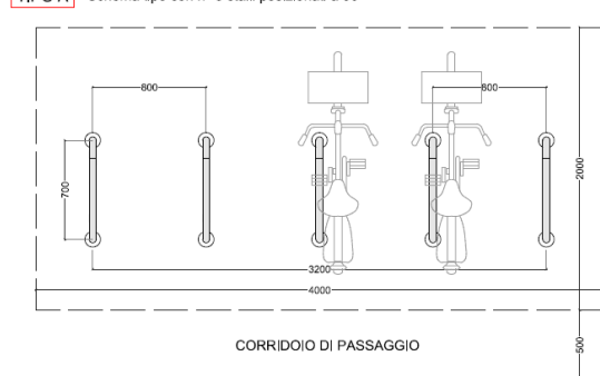
TIPO A Schema tipo con n° 5 stalli posizionati a 90°
